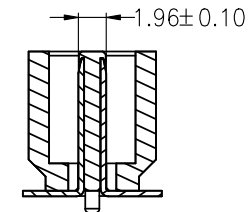
A-A SECTION
